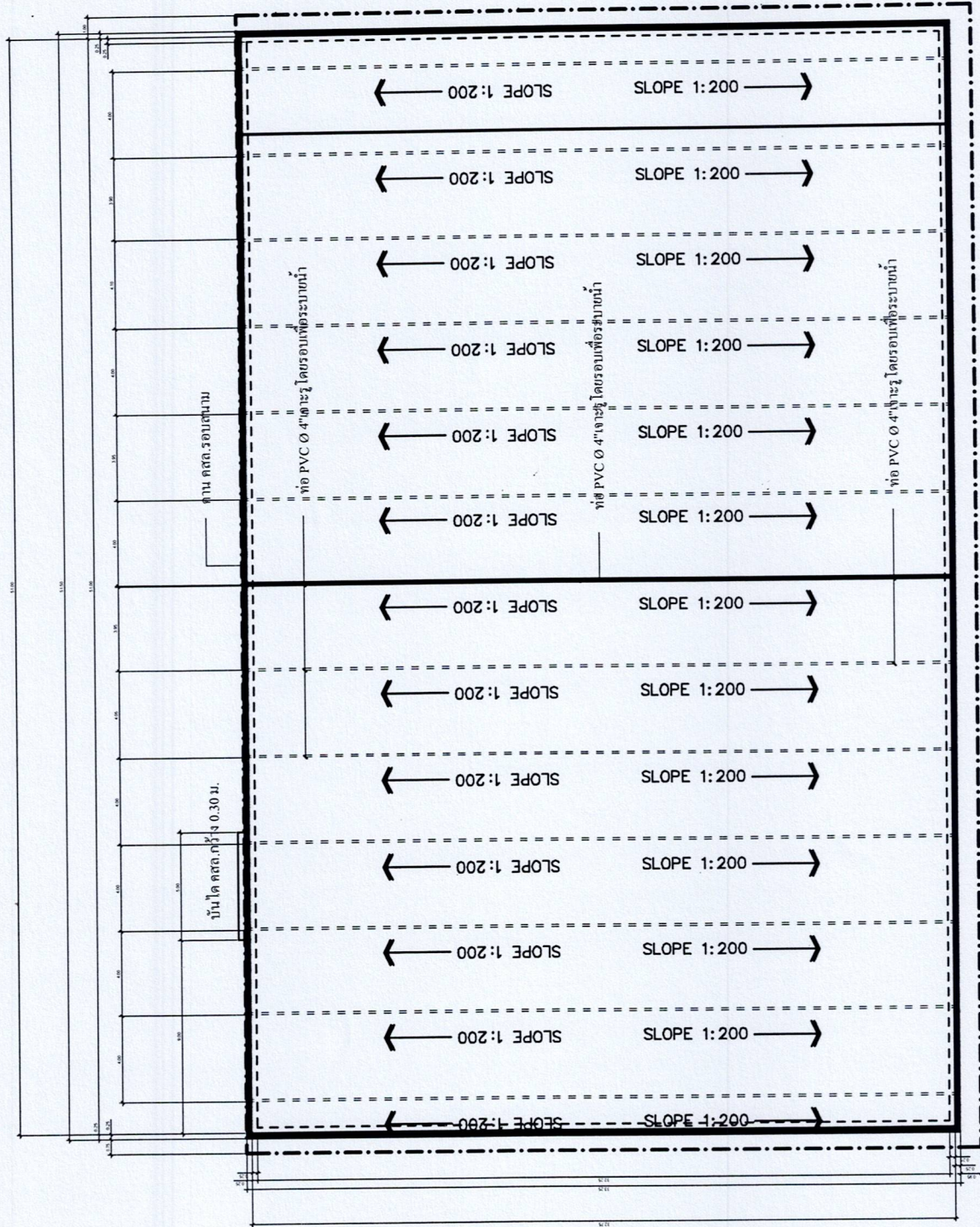
รูปแบบระบบระบายน้ำภายในสนามสนามฟุตชอยหน้าเทียบ
